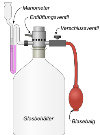
Abbildung 3: Skizze Clement-Desormes
